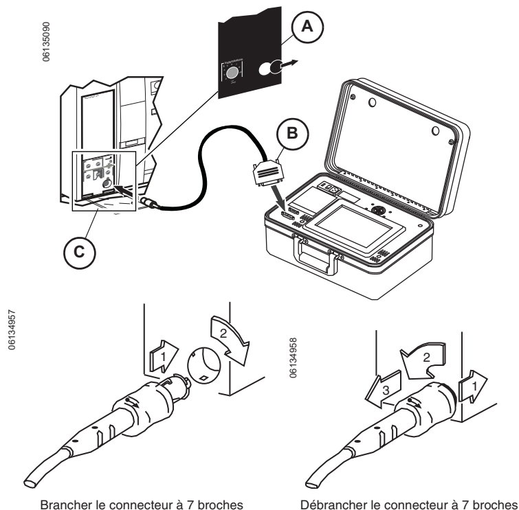
Figure 3 : Raccordement aux déclencheurs Micrologic et ET
